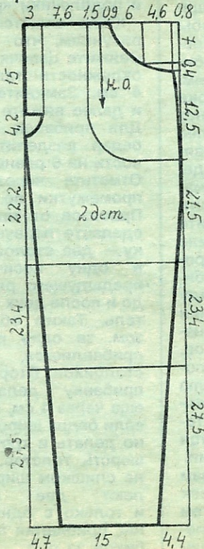
Передняя половинка брюк
