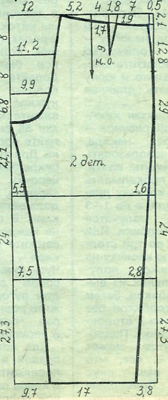
Задняя половинка брюк
