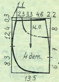
Деталь мешковины кармана
