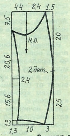
Задняя половинка брюк
